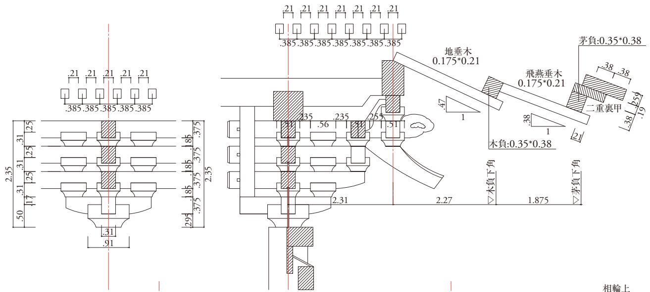
組物および軒先詳細図 縮尺:1/25(単位:尺)
