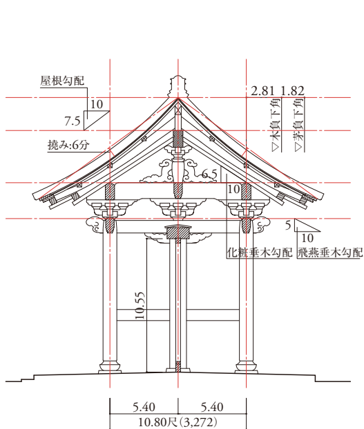
梁間・桁行 矩計図 縮尺:1/125(単位:尺)
