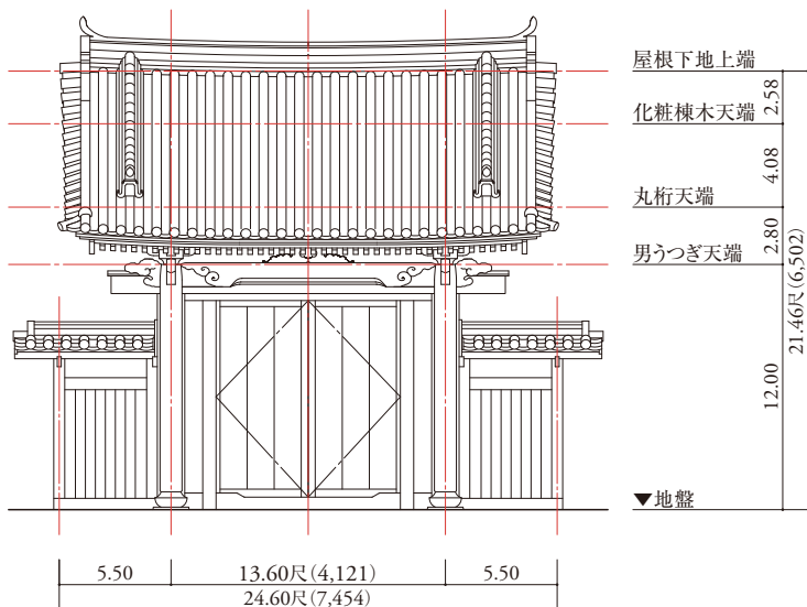
側面・正面 立面図 縮尺:1/125(単位:尺)
