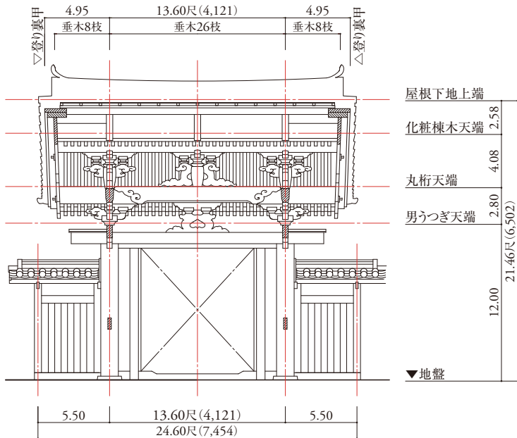
梁間・桁行 矩計図 縮尺:1/125(単位:尺)
