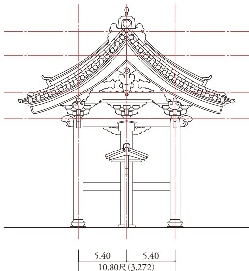
側面・正面 立面図 縮尺:1/125(単位:尺)
